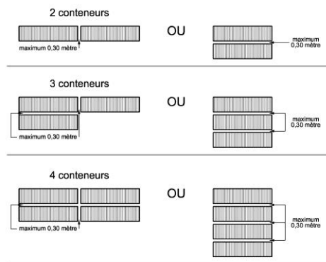
Croquis 7.1 Disposition des conteneurs
