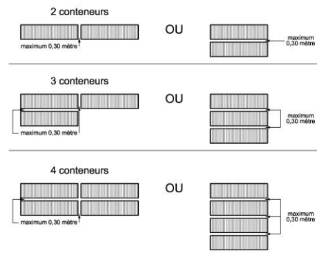
Croquis 7.1 Disposition des conteneurs
